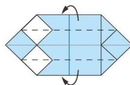
⓬ 沿虛線向後面摺
